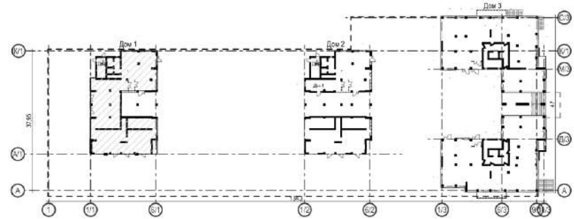
Компановочная схема
