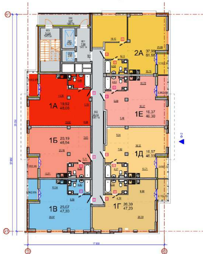
План типового этажа. Дом №2
